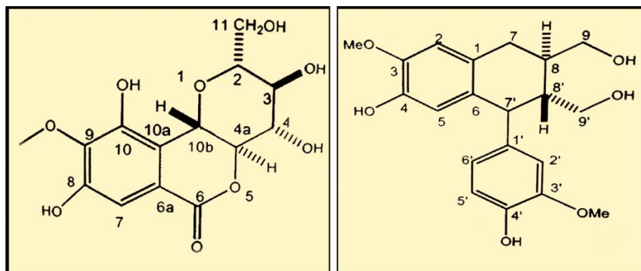
Bergenin
